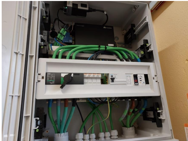
Cuadro Eléctrico
