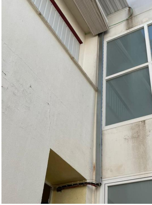
Cableado de conexión paneles fotovoltaicos a inversor
