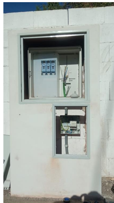
Módulo de Medida Edificio + Módulo de Medida Instalación Fotovoltaica Después
